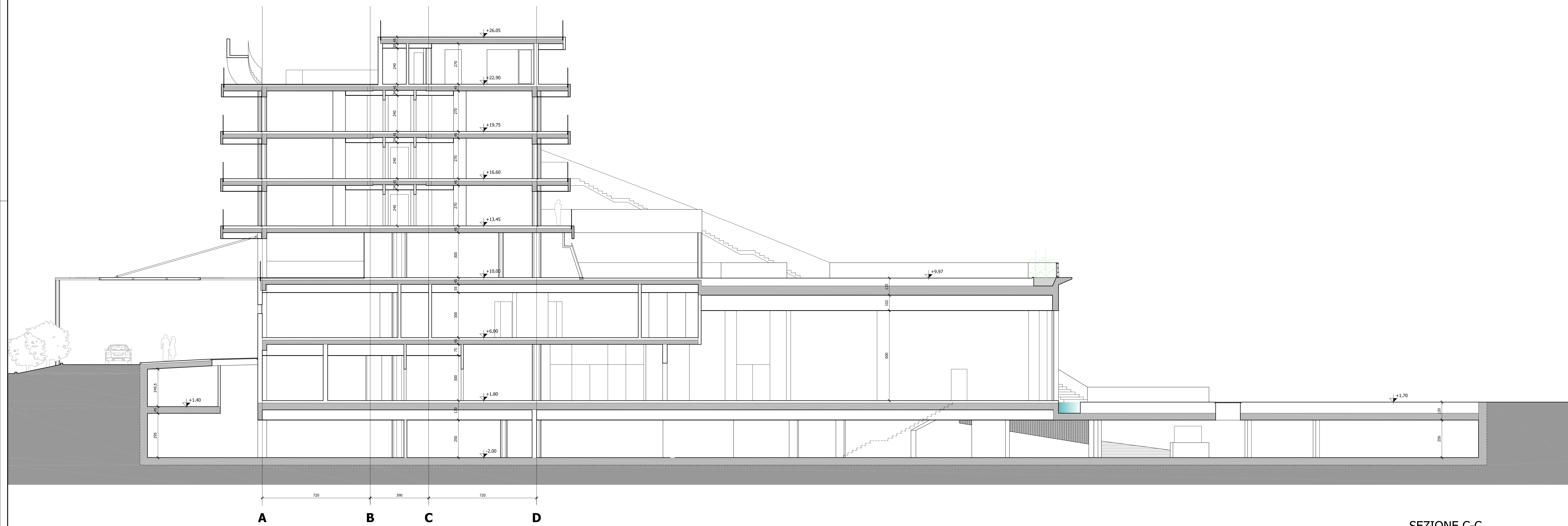
SEZIONE C-C
