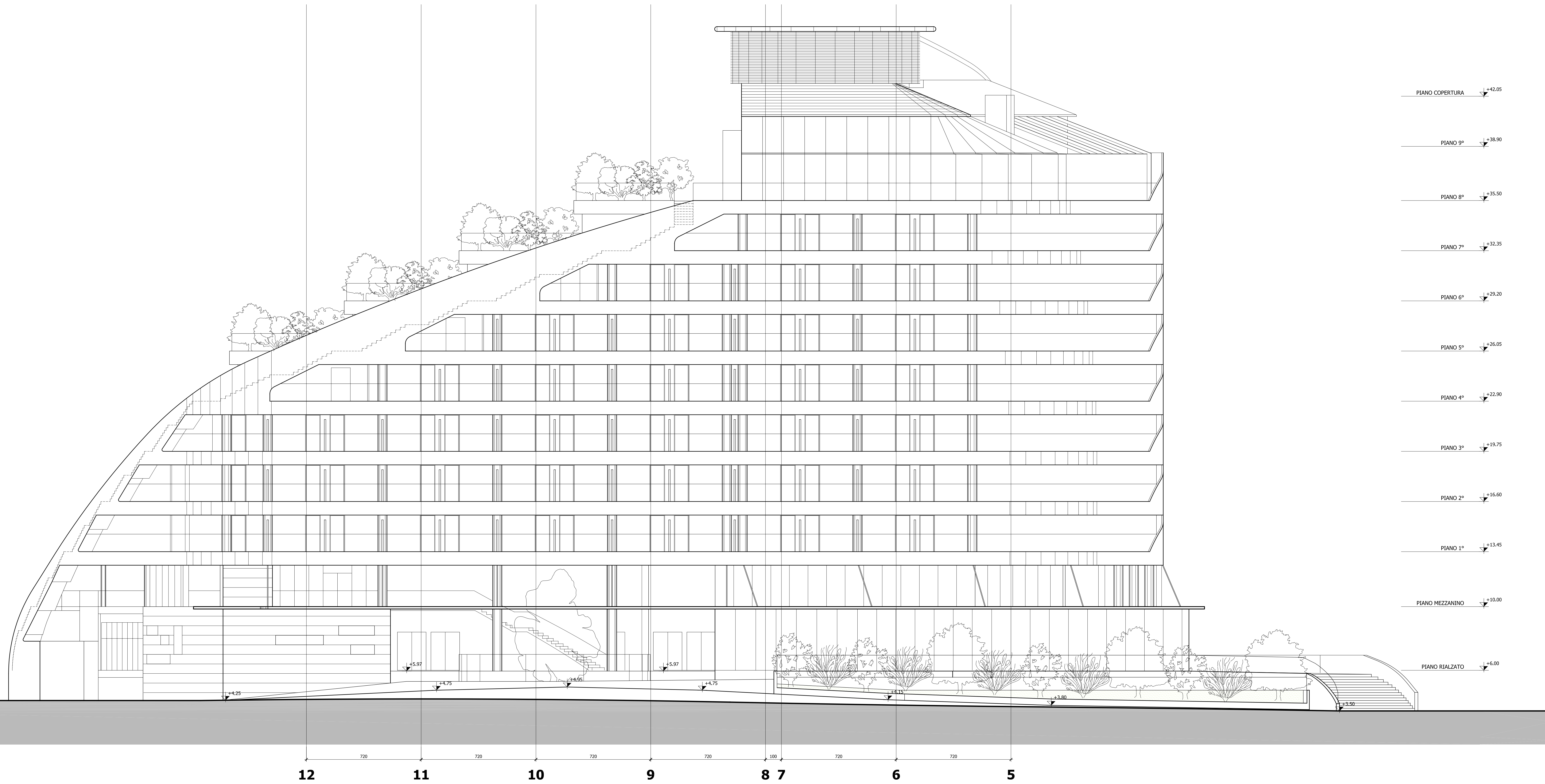
PROSPETTO NORD-EST
